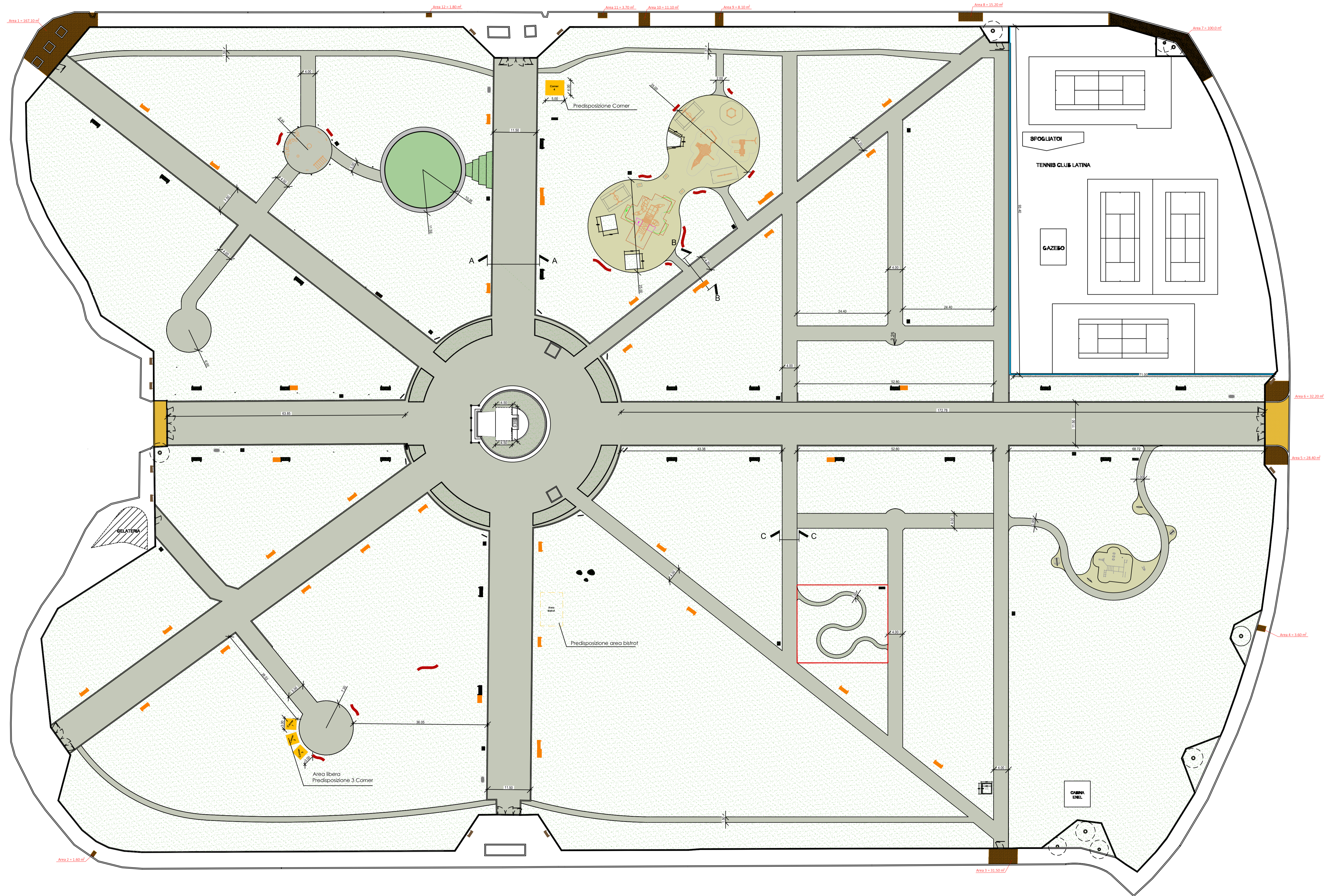
PLANIMETRIA GENERALE - INTERVENTO scala 1:500
